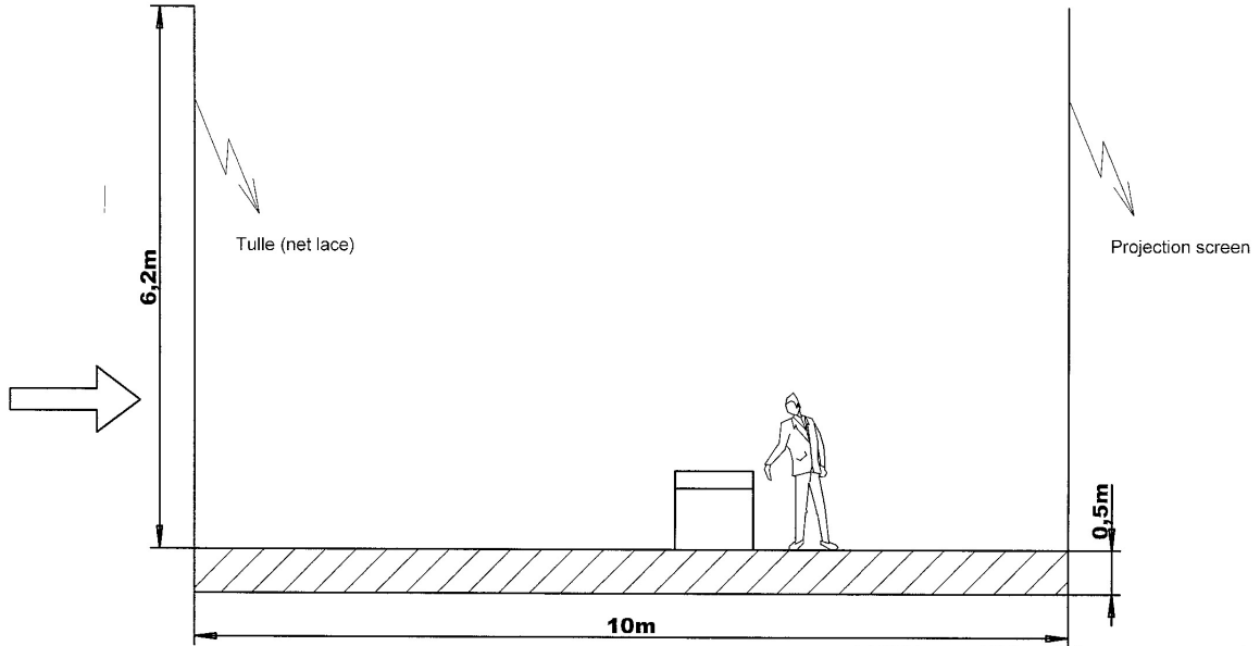
ITALIA ANNO ZERO Stage plan 1:50 LONGITUDINAL SECTION
